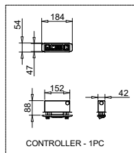
CONTROLLER - 1PC
